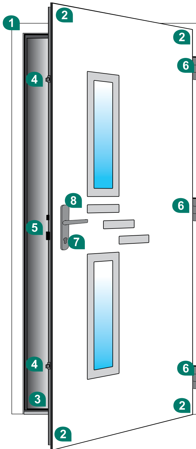
6 Paumelles cylindriques réglables en 3 dimensions Coloris standard : Titane Mat Autres coloris disponibles : (page 13)
