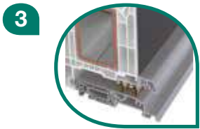
3 Seuil en aluminium avec barrière thermique (page 18)
