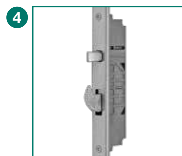
4 Système de fermeture type combi (gâche + crochet)
