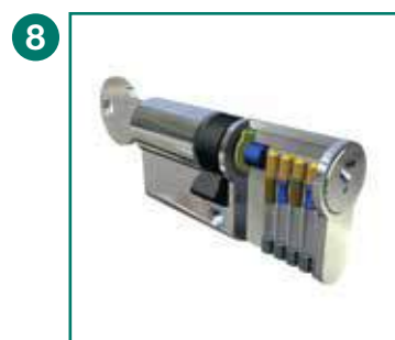
8 Cylindre argenté avec 5 clés
