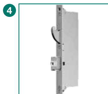
4 Point de fermeture à crochet avec verrouillage automatique
